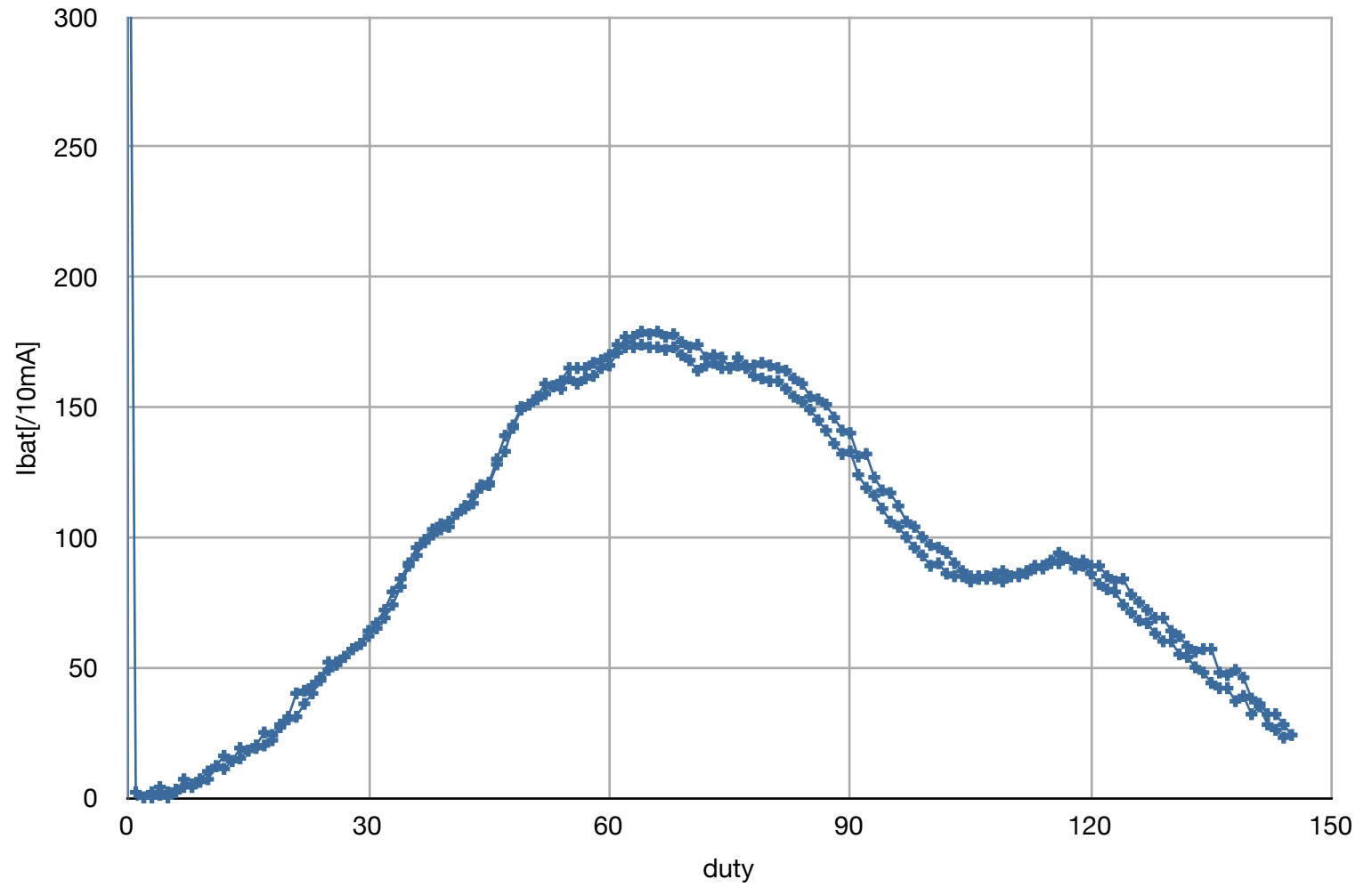
AKIZUKI-slim 100KHz
