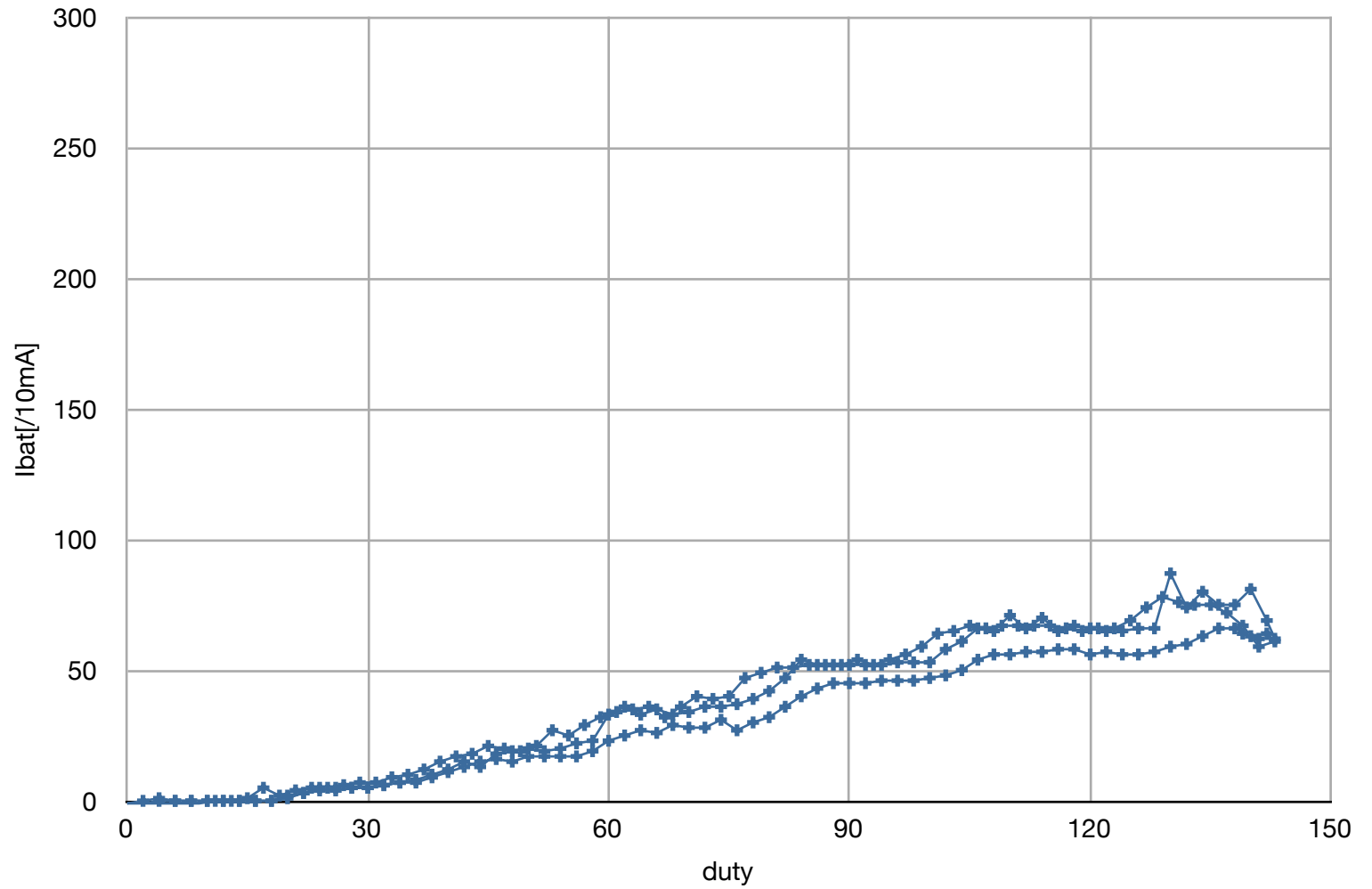
ETM250-1.5V#1 100KHz
