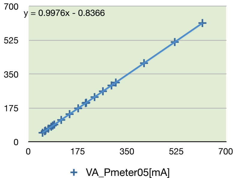
電流精度
