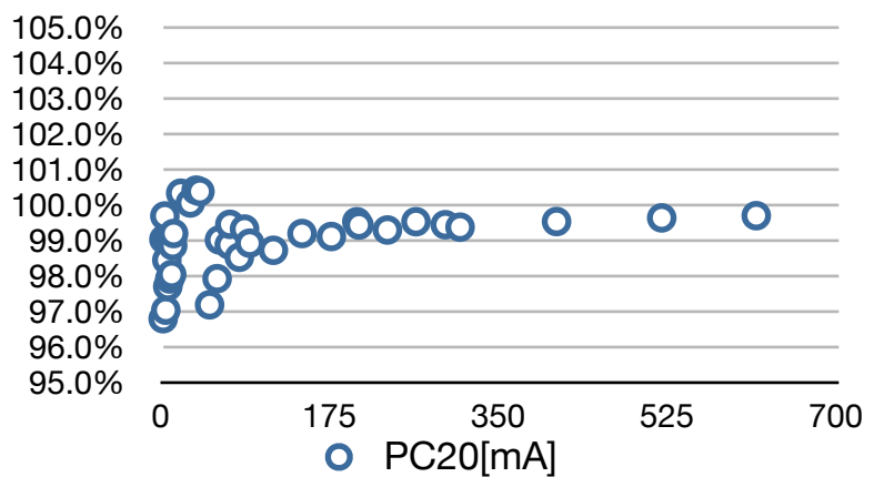
電流精度
